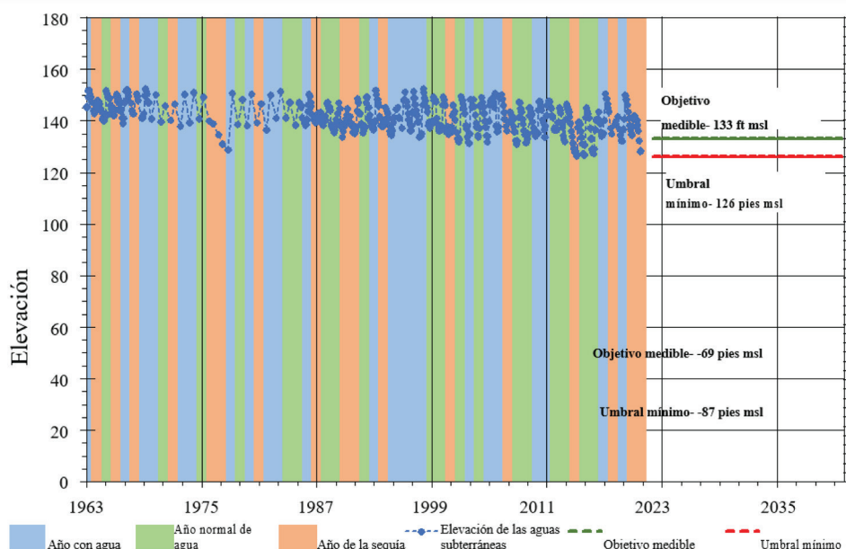
▲ Muestra de los datos de elevación de aguas subterráneas de pozo de monitoreo RMS
