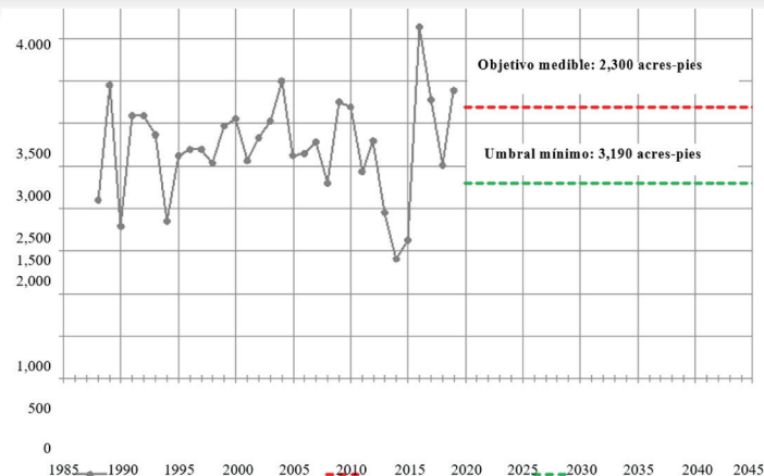
▲ Agotamiento estimado de las aguas superficiales debido a la extracción de agua subterránea en el río Napa, cerca de Napa
