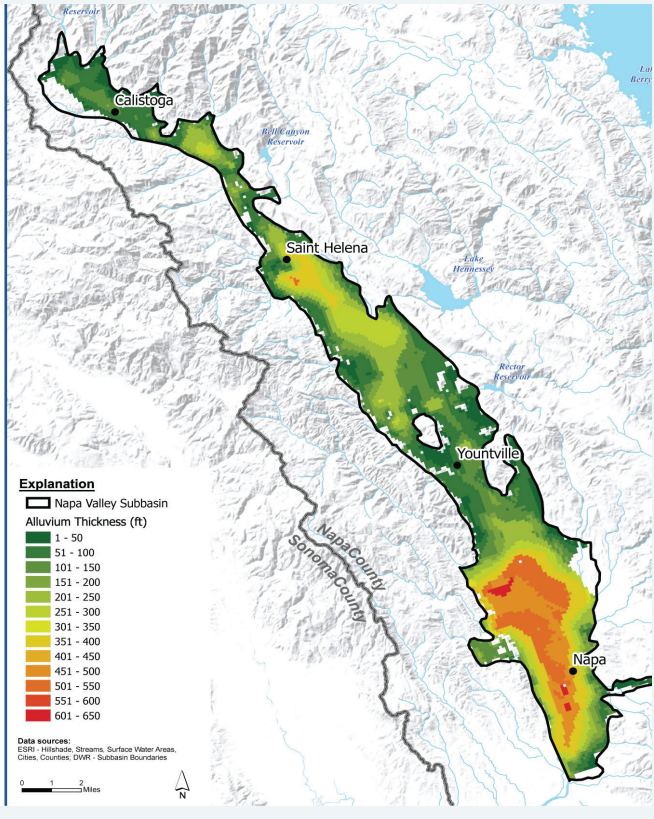
▲ Espesor del aluvión cuaternario
