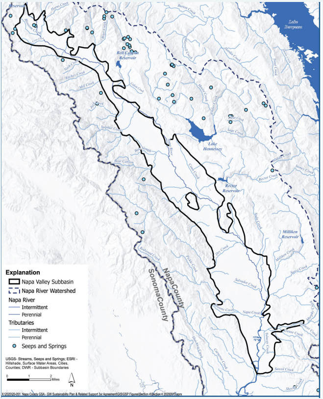
▲ Características de las aguas superficiales y los humedales
